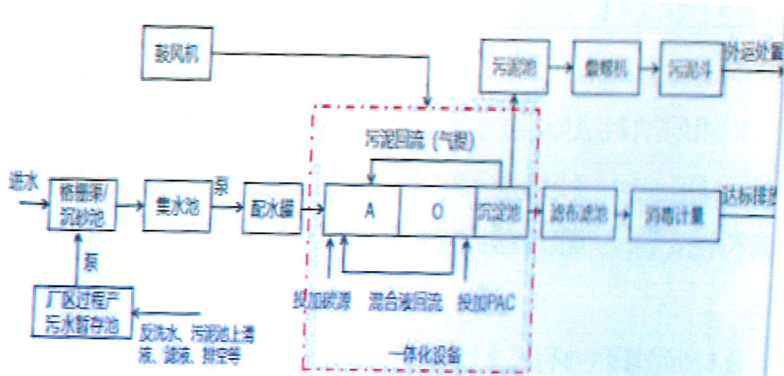
图 4-1 本项目污水处理工艺流程图
